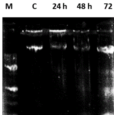
شکل ۳. اثرات ترکیب 2-DP.P بر قطعه قطعه شدن DNA در سلول های K562. سلول ها با ترکیب مورد نظر در غلظت ۲۵ میکرومولار به مدت ۲۴، ۴۸ و ۷۲ ساعت تیمار شدند و اثرات آپوپتوزی به وسیله ی قطعه قطعه شدن DNA با استفاده از الکتروفورز ژل آگارز بررسی گردید. M: ladder marker ، C: نمونه ی کنترل
